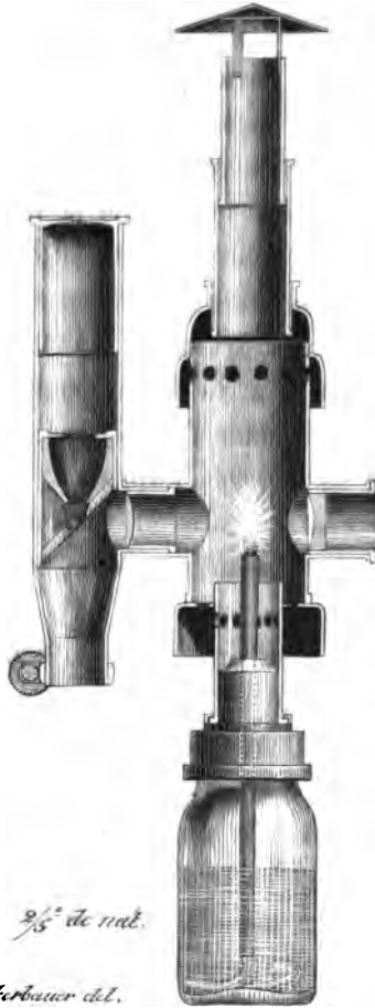
Fig. 2. — Coupe de l'endoscope.
